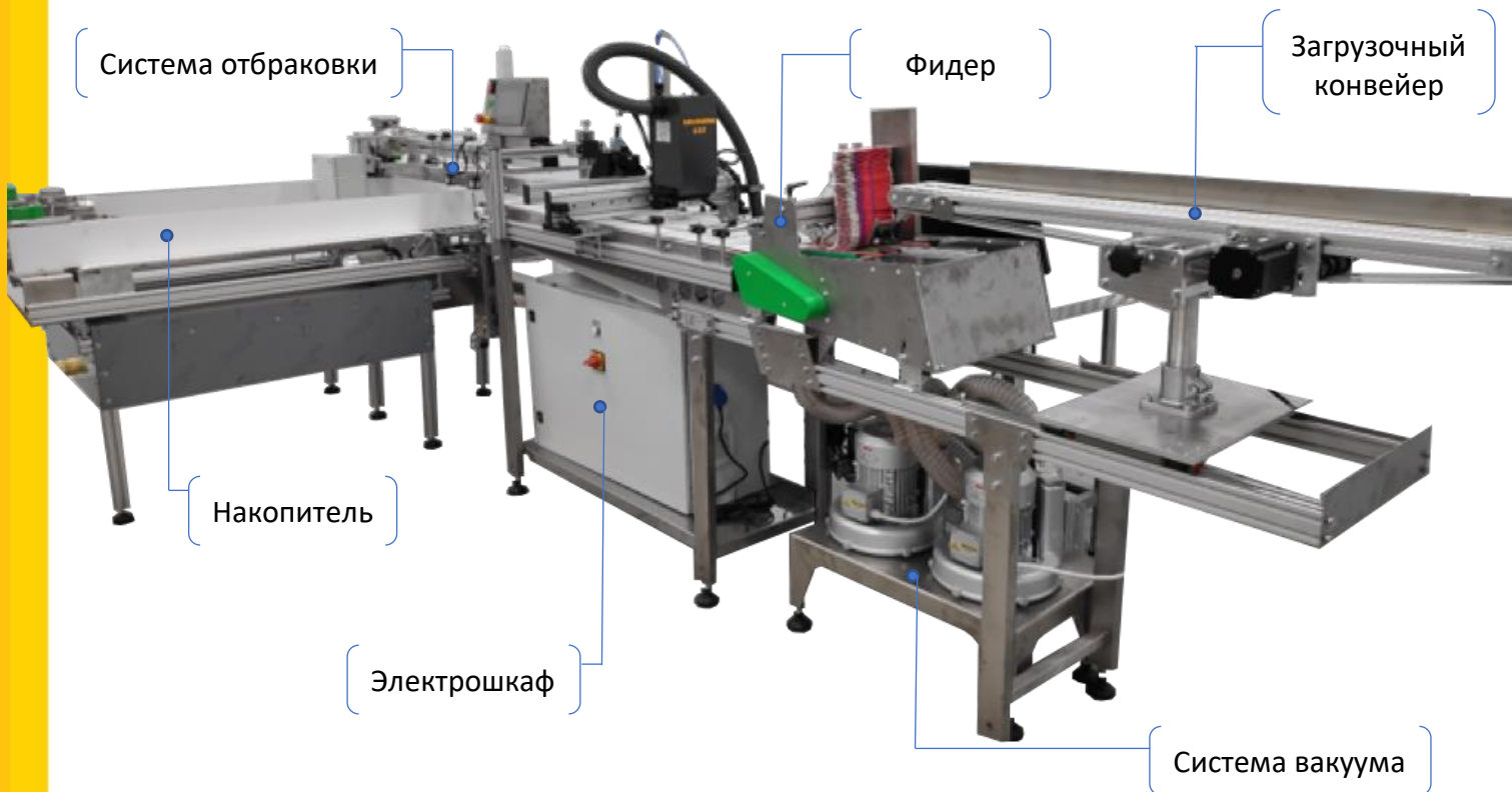
Загрузочный конвейер для подачи плоских пачек в пролистыватель
