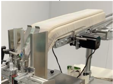
Загрузочный конвейер для подачи плоских пачек в пролистыватель
