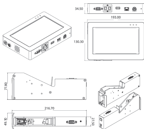
Габаритные размеры Solmark S20 MAX (контроллер и печатная головка)
