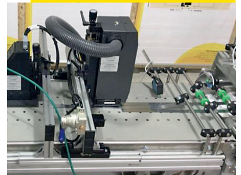
Вакуумный конвейер
