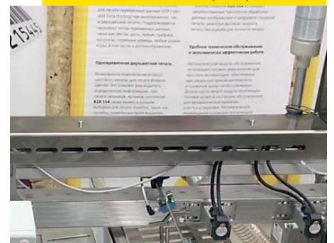
Система отбраковки с сервоприводом
